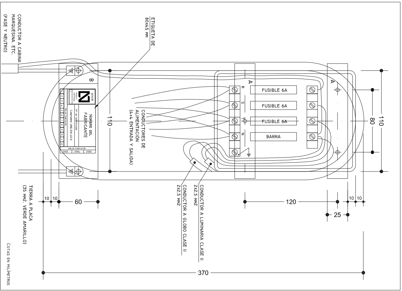
ESQUEMA DE CONEXIONADO EN BACULO Y COLUMNA DE 8 A 18 M. DE ALTURA
