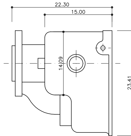
ALZADO LATERAL
