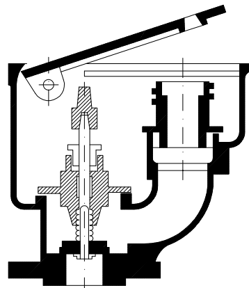
SECCION
