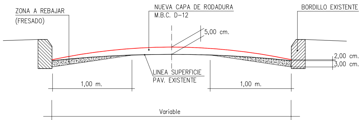
SECCIÓN TIPO
