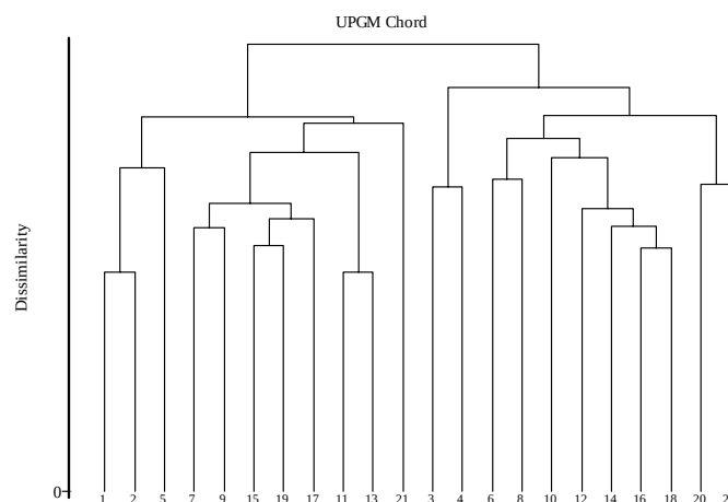
Figura. 10. Clasificación jerárquica utilizando la distancia de la cuerda (chord distance) para calcular la matriz de semejanzas, y "Unweighted Pair-Group Methods using Arithmetic Averages" en el proceso de aglomeración.
