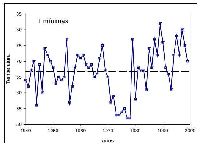
Gráfico 4: Evolución de las temperaturas mínimas en el periodo 1940-1999. Elaboración a partir de datos de la estación meteorológica de Mora.
