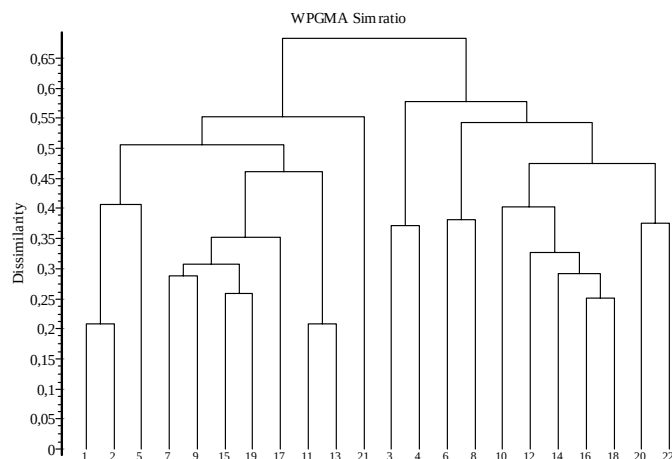
Figura. 11. Clasificación jerárquica utilizando la distancia de la proporción de semejanza (similarity ratio) para calcular la matriz de semejanzas, y “Weighted Pair-Group Methods using Arithmetic Averages” en el proceso de aglomeración.
