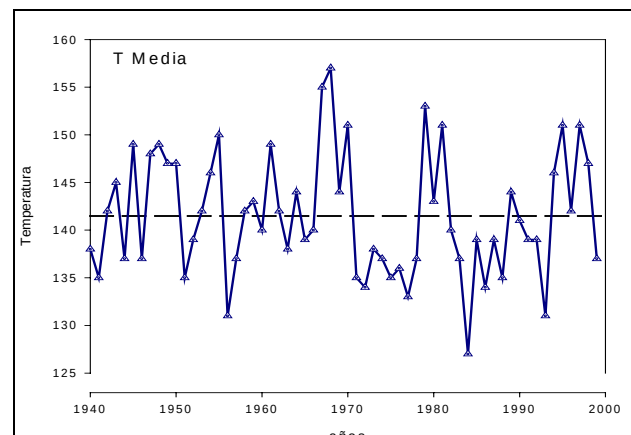
Gráfico 3: Evolución de las temperaturas medias en el periodo 1940-1999. Elaboración a partir de datos de la estación meteorológica de Mora.
