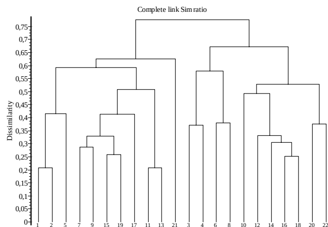
Figura. 9. Clasificación jerárquica utilizando la proporción de semejanza (similarity ratio) para calcular la matriz de semejanzas, y vinculación completa (complete linkage) en el proceso de aglomeración.
