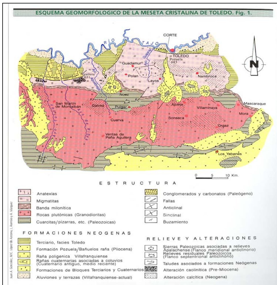
Figura 2: Esquema geomorfológico de la Meseta Cristalina de Toledo (Vázquez González, Asensio Amor, González Martín 1998). Guía de Espacios Protegidos de Castilla la Mancha, pag 386).
