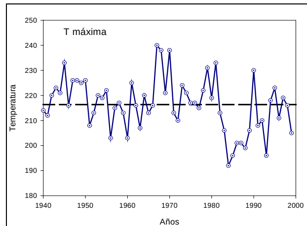
Gráfico 2: Evolución de las temperaturas máximas 1940-1999. Elaboración a partir de datos de la estación meteorológica de Mora. (Los datos de temperatura se dan en C° multiplicados por 10 para facilitar su manejo)
