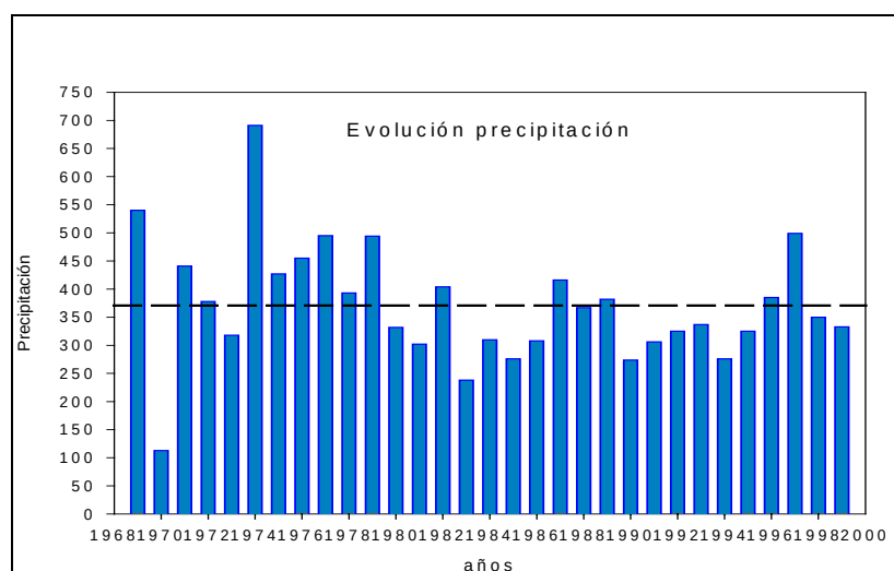
Gráfico 5: Datos de precipitación de la estación meteorológica de Mora en el periodo 1969-1999.
