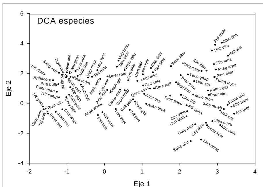
Figura 13. Representación del DCA especies.
