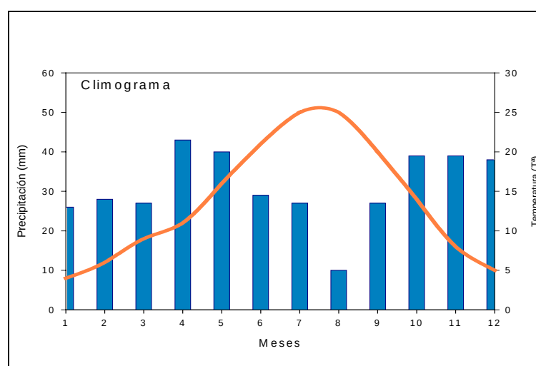
Gráfico 1: Climograma (Elaboración a partir de datos de la Estación meteorológica de Mora).
